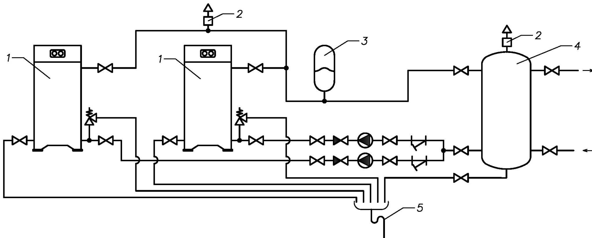
Рис. 8 Упрощенная схема подключения водонагревателя в систему водоснабжения.
